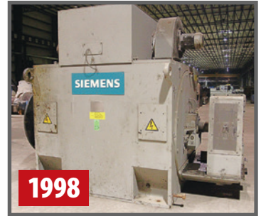
6623 KW SIEMENS 1DQ3843-6 BD 03-Z MOTOR
