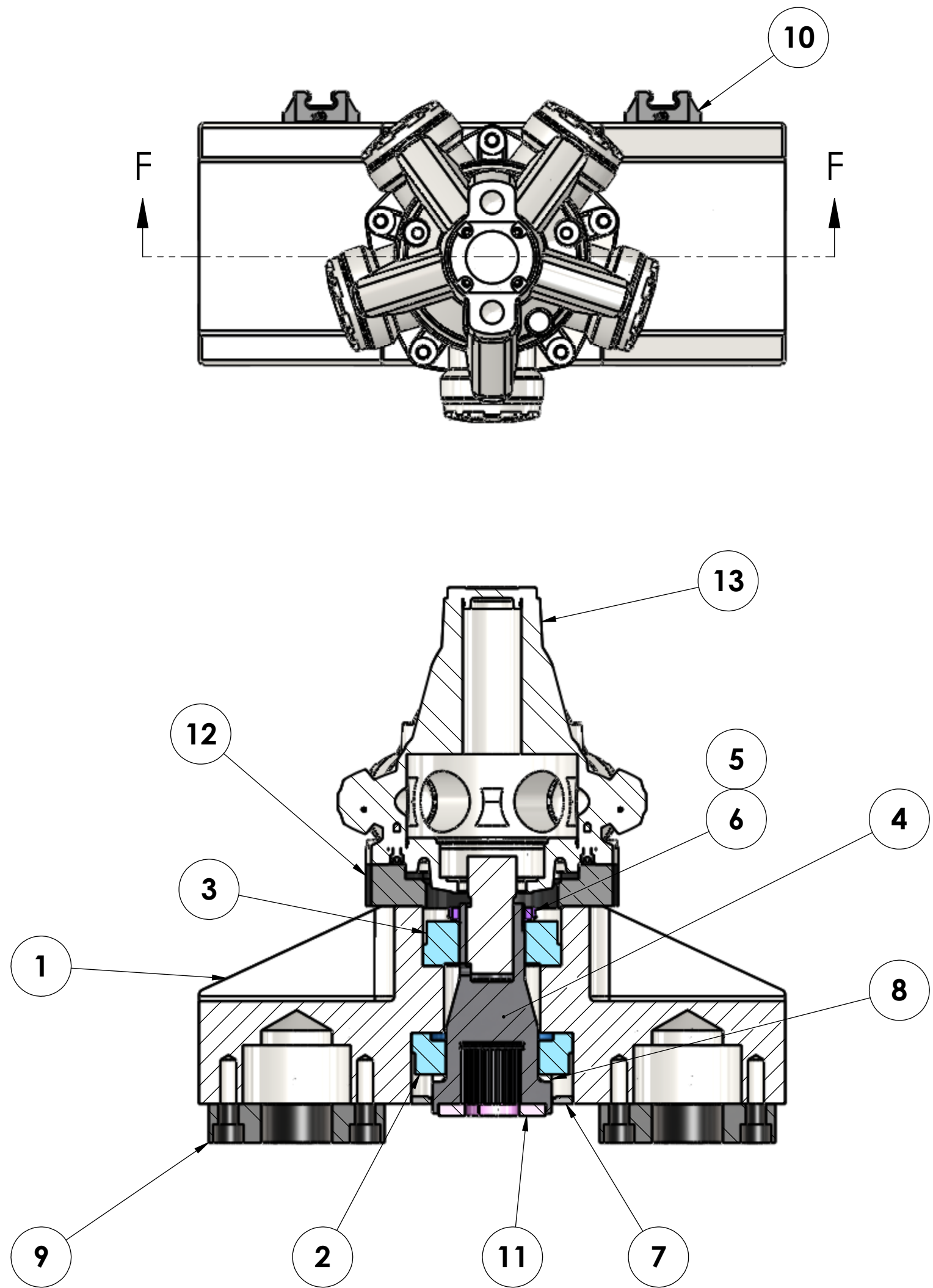
SECTION F-F SCALE 1 : 6
