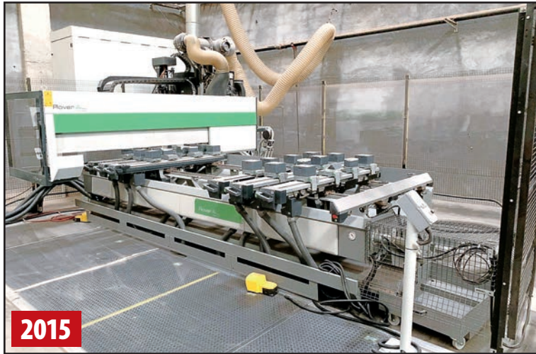
Centro de maquinado CNC para fresar y pegar chapa en los cantos de tableros de madera, Biesse Rover A Edge 1632
